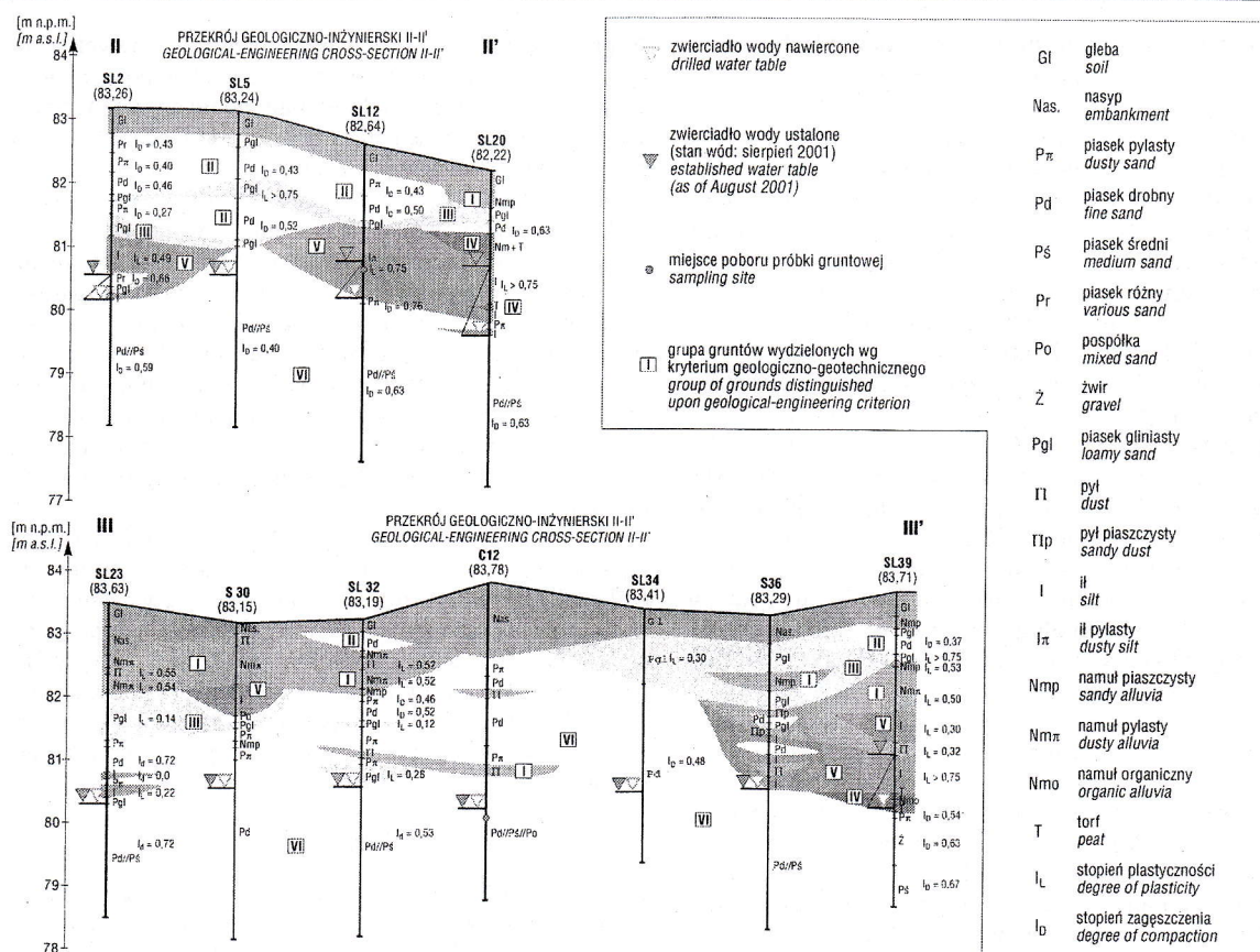
Ryc. 2. Przekroje geologiczno-inżynierskie Fig. 2. Geological and engineering cross-sections
